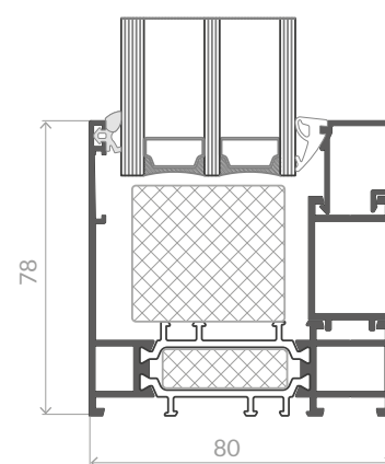
Řez pevného dílu okna se skrytým křídlem
