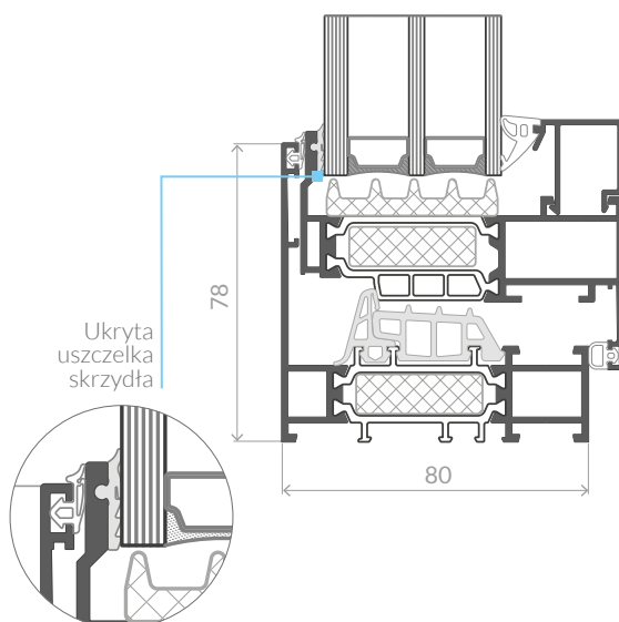
Řez otevíravého okna se skrytým křídlem
