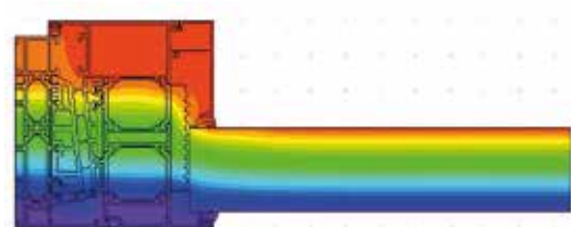
Rozložení teplot
