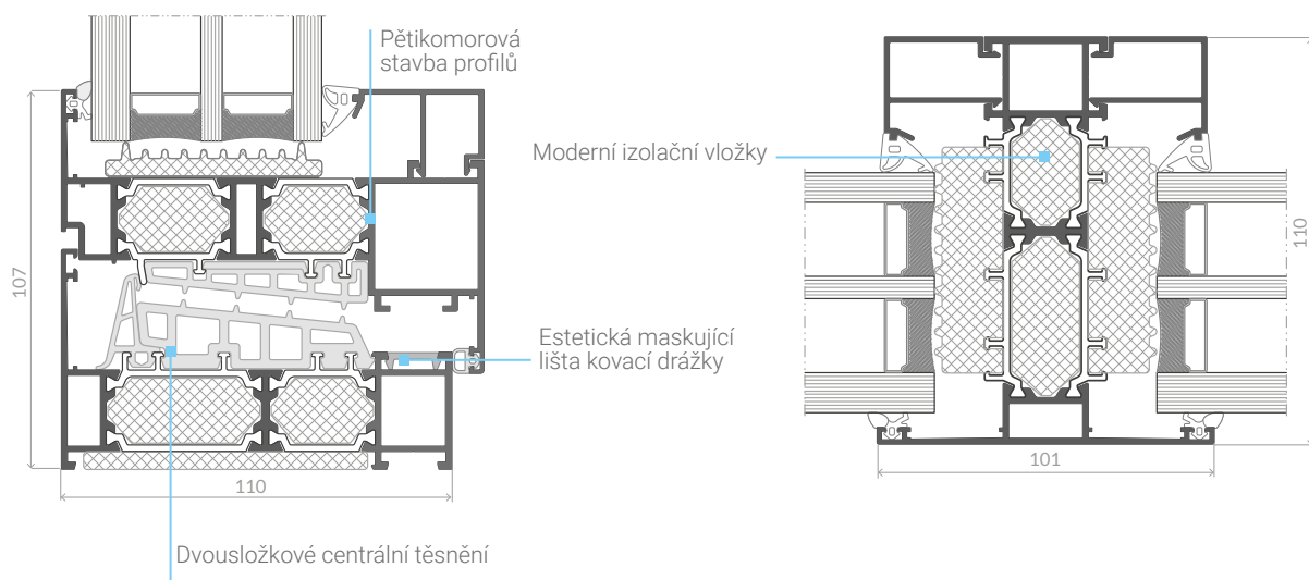
Řez otevíravým oknem
